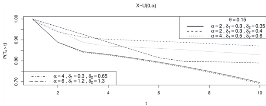
شکل (۳): عملکرد تابع بقاء سیستم در توزیع یکنواخت به ازای \alpha = 2, 4, 6 ، \delta_1 = 0/3, 0/5, 1/2 و \delta_2 = 0/35, 0/4, 0/65, 1/3, 1/3
