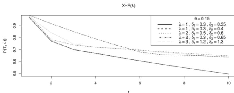
شکل (۶): عملکرد تابع بقاء سیستم در توزیع نمایی به ازای \theta = 0.15 ، \delta_1 = 0.3, 0.5, 1.2 و \delta_2 = 0.35, 0.4, 0.6, 0.65, 1.3 و \lambda = 1, 2, 3
