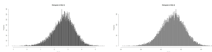
شکل ۸: توزیع برآوردگرهای \vec{\beta}_0 = (\hat{\beta}_0, \hat{\gamma}_0, \hat{\theta}_0)
