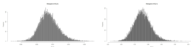
شکل ۹: توزیع برآوردگرهای \vec{\beta}_1 = (\hat{\beta}_1, \hat{\gamma}_1, \hat{\theta}_1)
