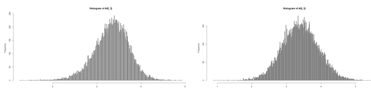
شکل ۵: توزیع برآوردگرهای \vec{\Xi}_0 = (\hat{\beta}_0, \hat{\gamma}_0, \hat{\theta}_0) به ترتیب از چپ به راست برای \hat{\gamma}_0 و \hat{\theta}_0 .
